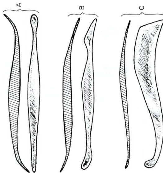
Một số kiểu bay nặn bằng gỗ, đôn hoặc thép, inox (mặt cắt bên trên, mặt chính diện bên dưới)
